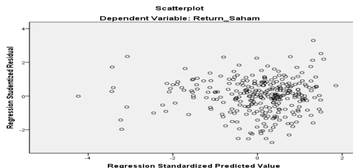
Gambar 5 Uji Heteroskedastisitas
