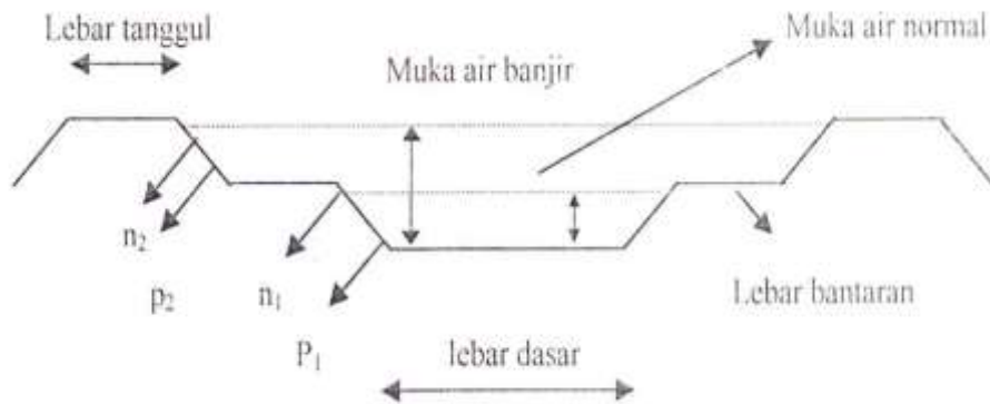
Gambar 2. 1. Sketsa Penampang Majemuk
