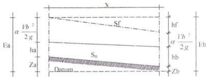
Gambar 3.2. Analisa perhitungan kedalaman kritis
