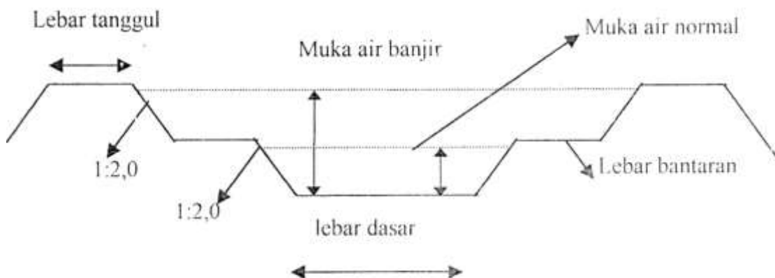
Gambar 2.3. Penampang Rencana
