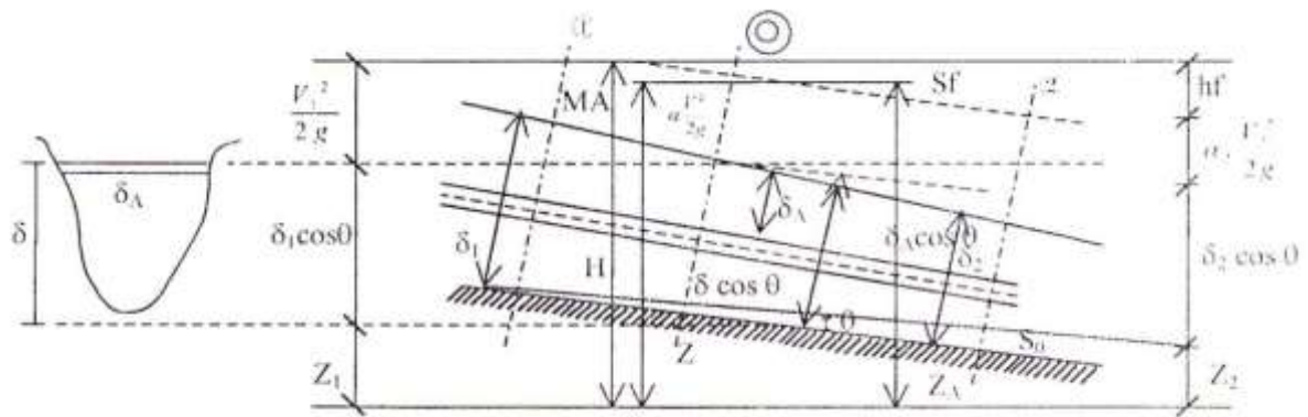
Gambar 3.1. Analisa Aliran Dengan Metode Standar Step
