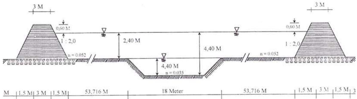
Gambar 3.4. Dimensi Penampang
