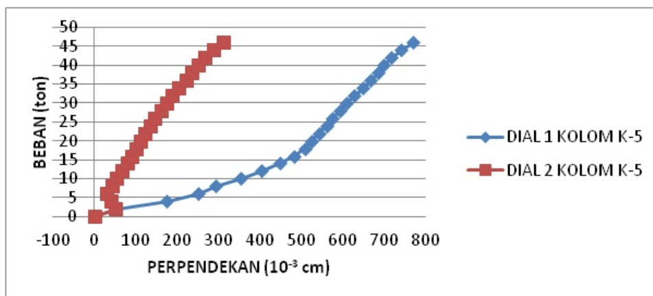
Gambar 11. Grafik hubungan beban dan perpendekan kolom K-5
