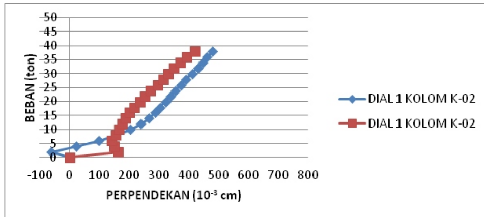
Gambar 10. Grafik hubungan beban dan perpendekan kolom K-02
