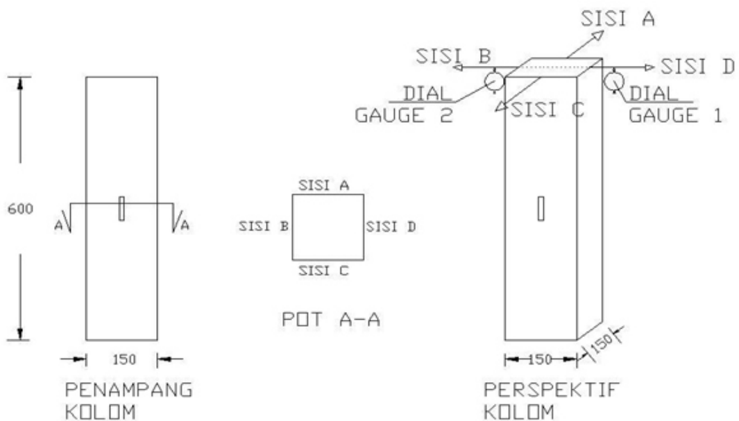
Gambar 3. Setting-up dial-gauge untuk mengukur perpendekan kolom
