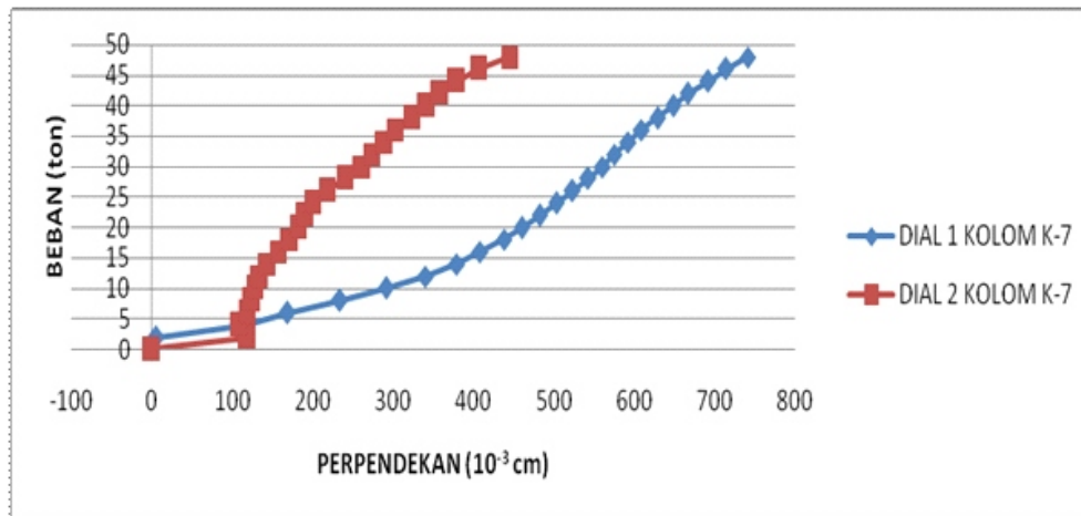
Gambar 12. Grafik hubungan beban dan perpindahan kolom K-7
