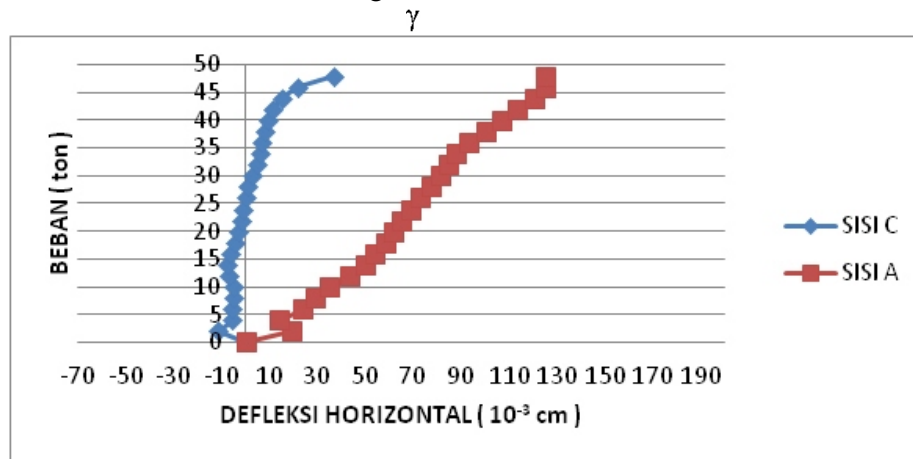
Gambar 7. Grafik hubungan beban dan defleksi lateral kolom K-5
