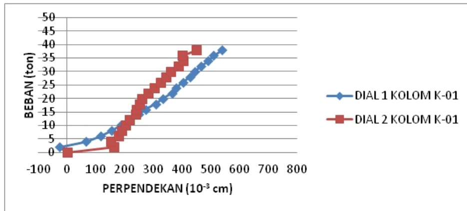
Gambar 9. Grafik hubungan beban dan perpendekan kolom K-01
